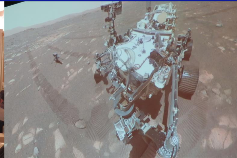
火星探査車 「パーサヴィアランス」
